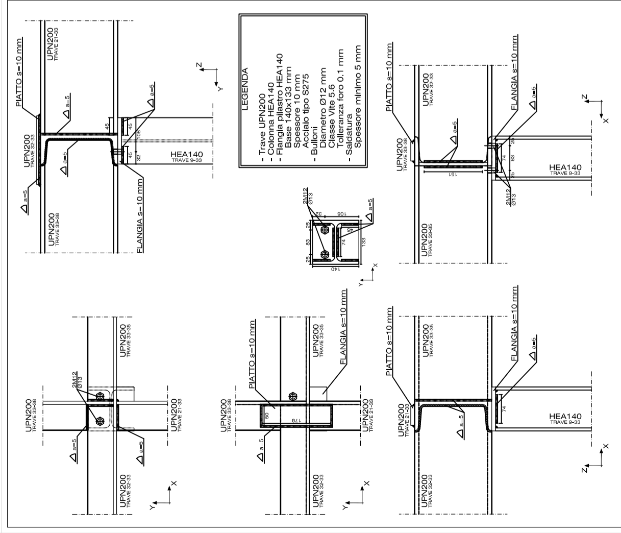
PARTICOLARE NODI: 33
