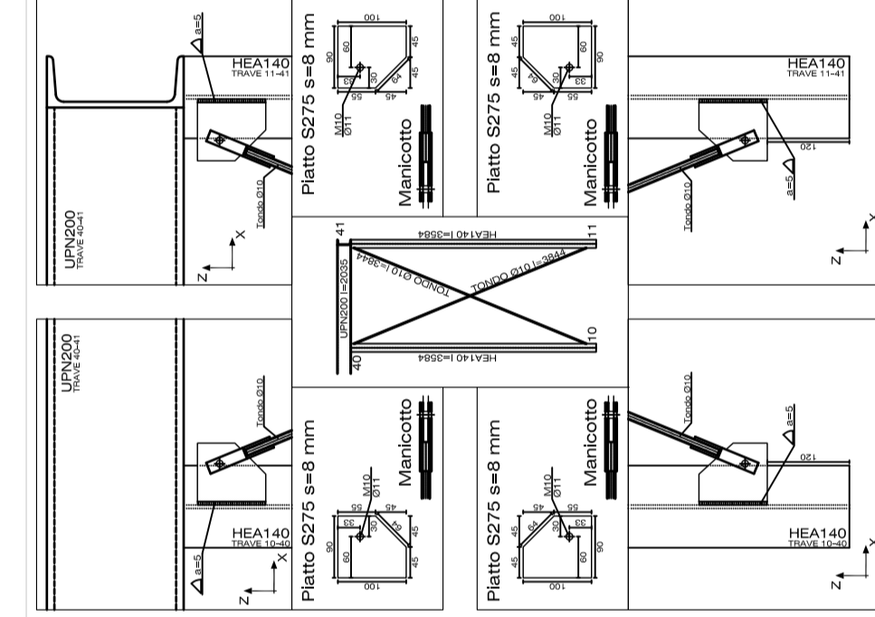
PARTICOLARE NODI: 10 - 11 - 40 - 41
