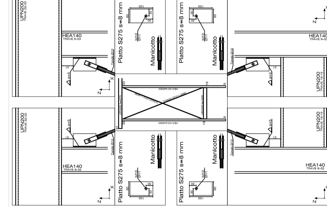
PARTICOLARE NODI: 18 - 43 - 32 - 33
